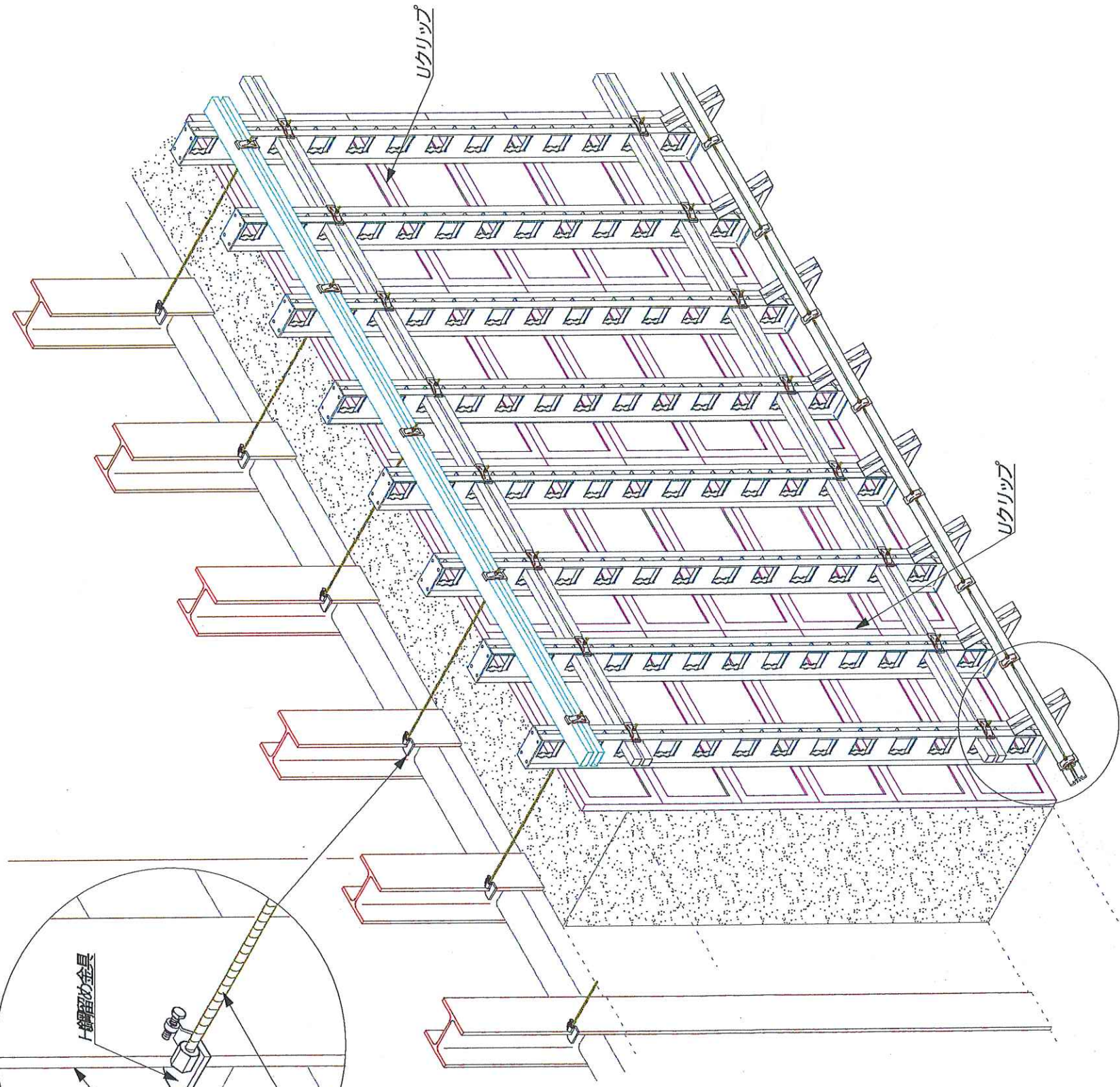
脚元詳細図
