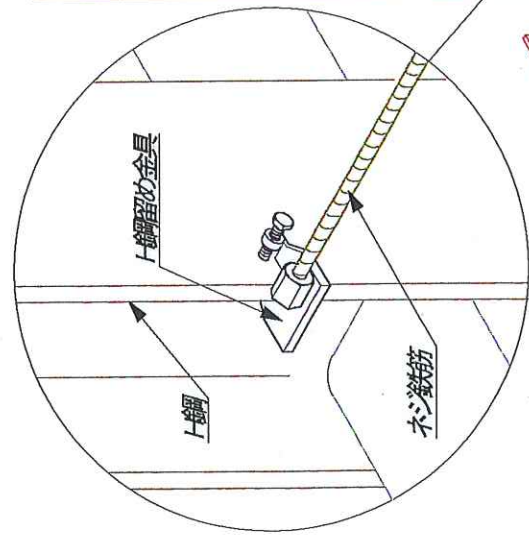
金具詳細図
